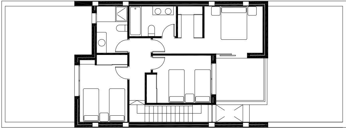
PLANTA PRIMERA
